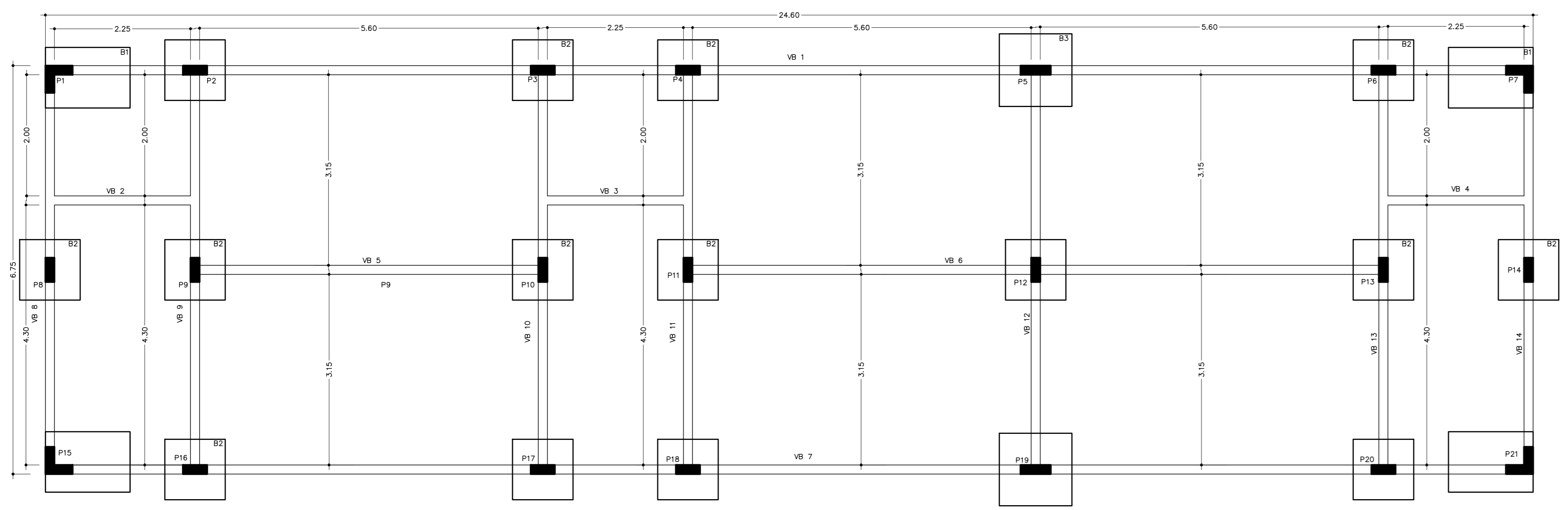
PLANTA DE LOCAÇÃO VIGAS BALDRAMES Escala: 1/20
