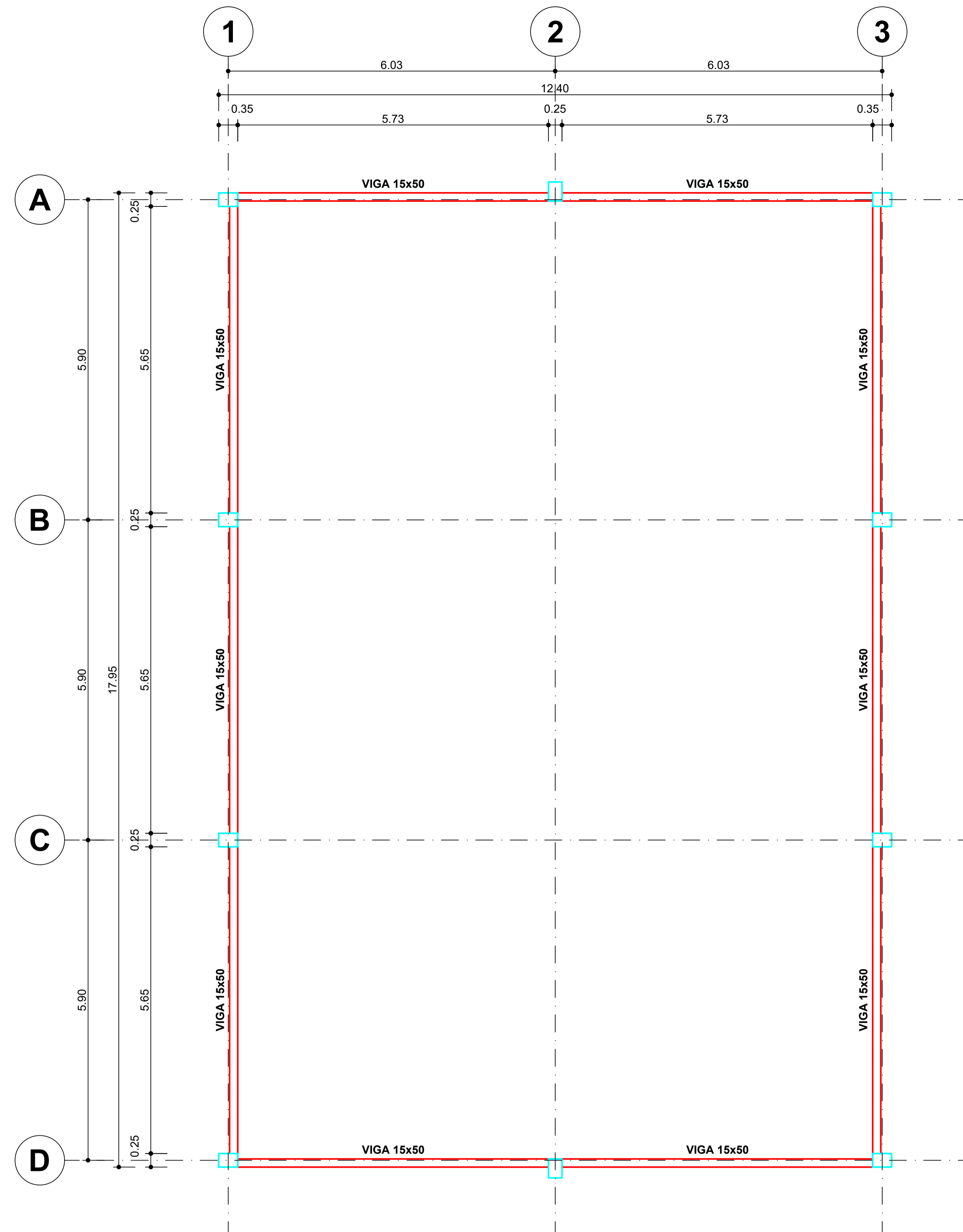
PLANTA DE FORMA - NÍVEL +0,00 ESCALA: 1/50
