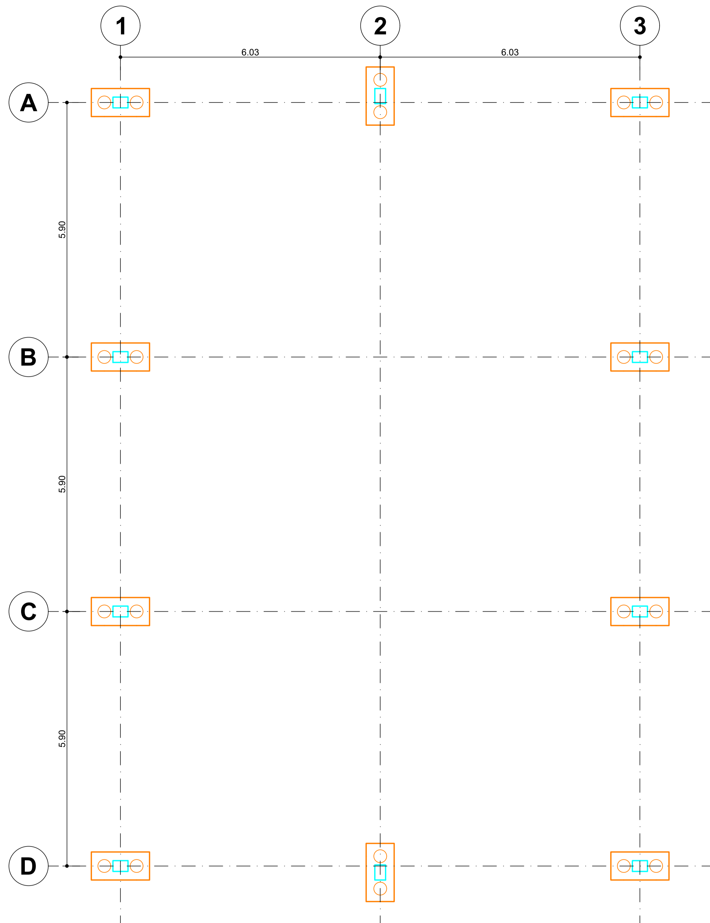
LOCAÇÃO ESCALA: 1/50
