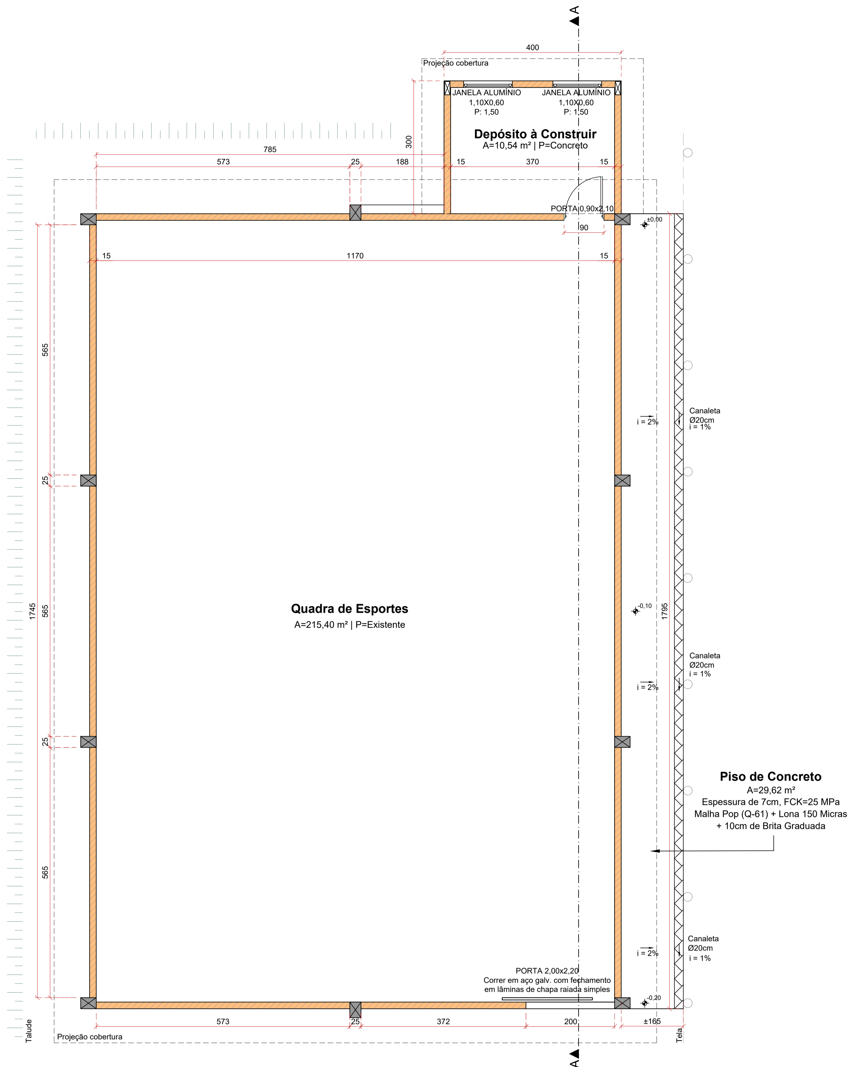
PLANTA BAIXA ESC.: 1/50
