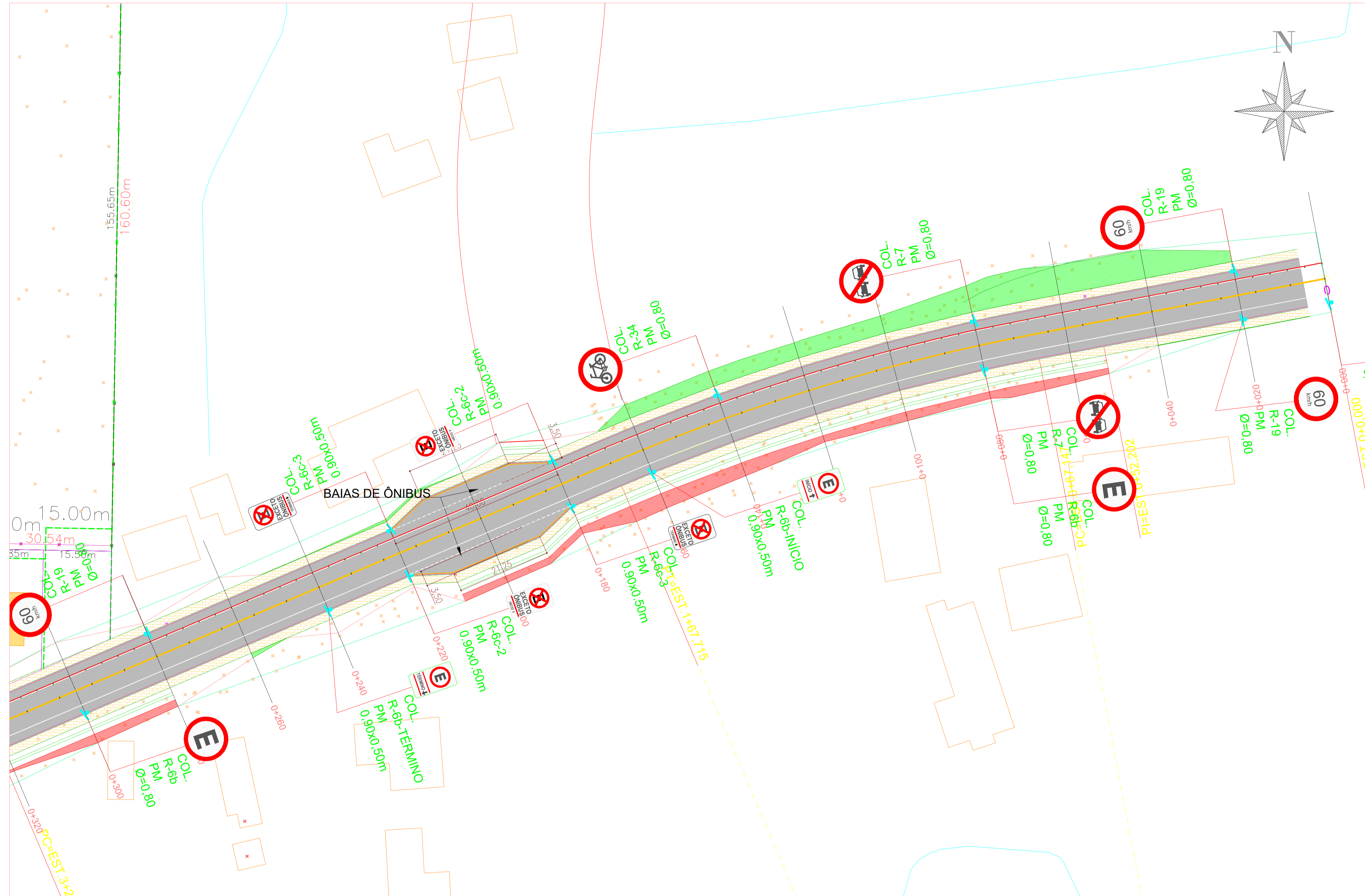
PLANTA BAIXA ESTACA 0+000 A 0+300 ESC: 1/500
