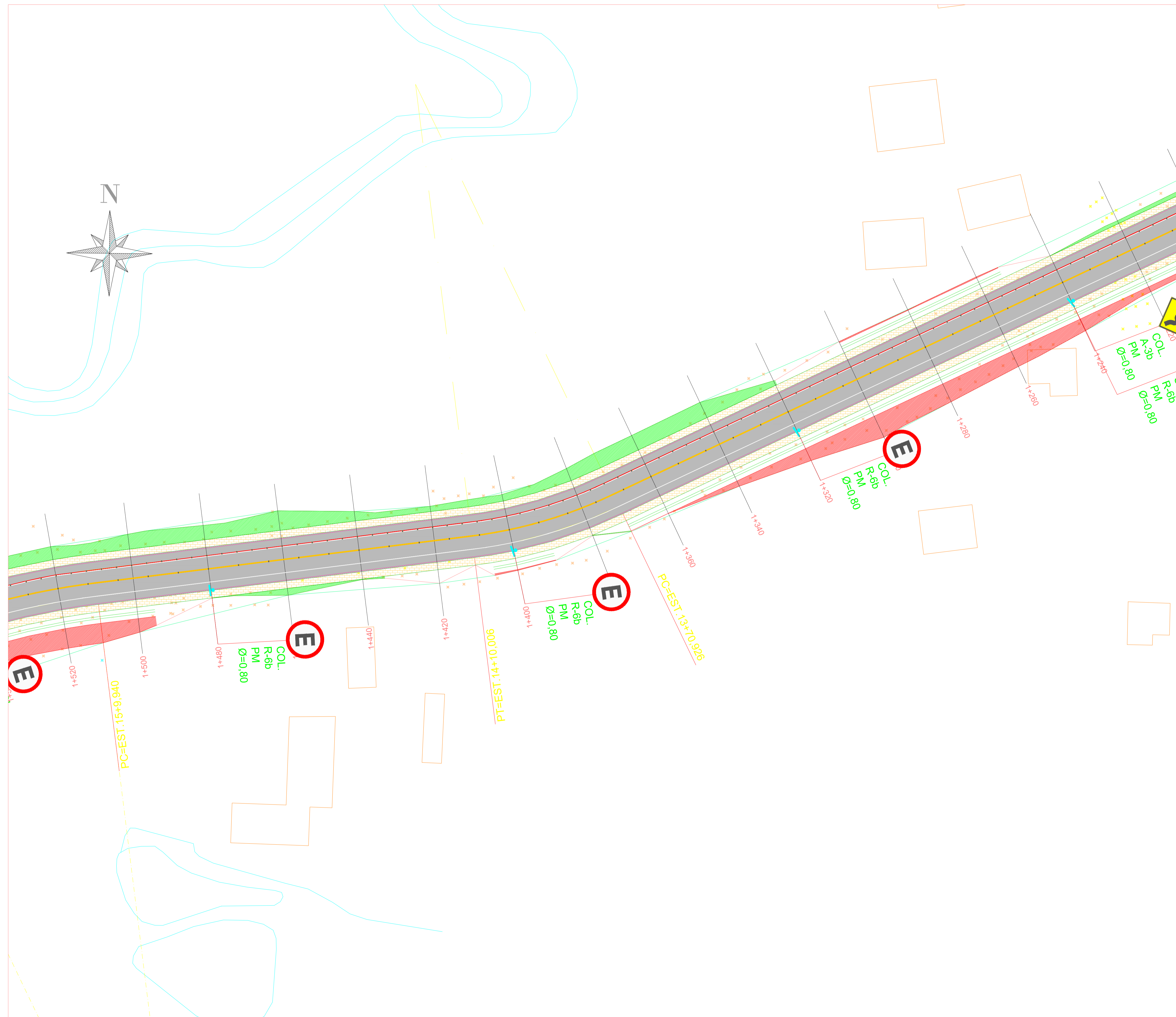
PLANTA BAIXA ESTACA 1+220 A 1+520 ESC: 1/500
