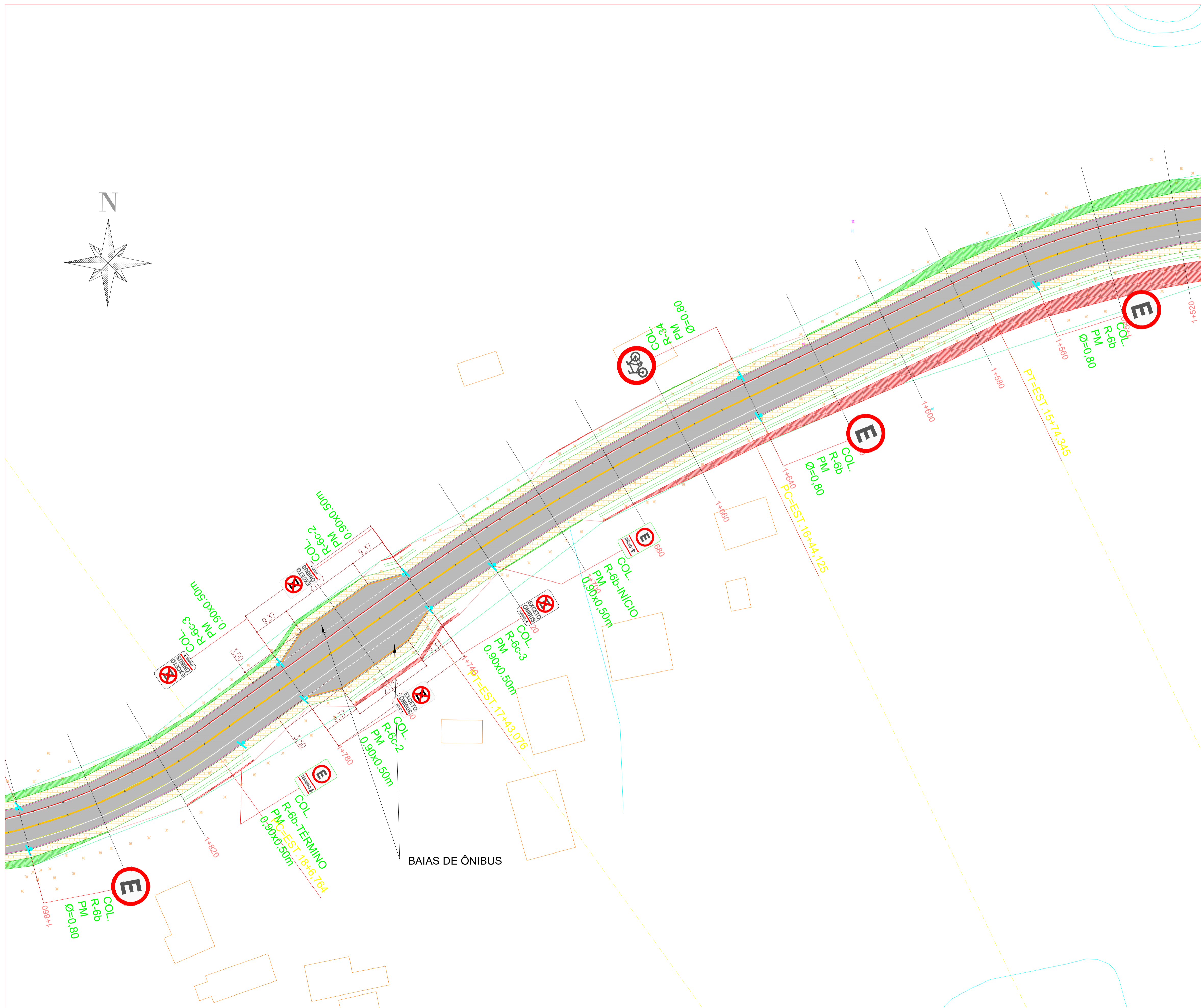
PLANTA BAIXA ESTACA 1+520 A 1+860 ESC: 1/500
