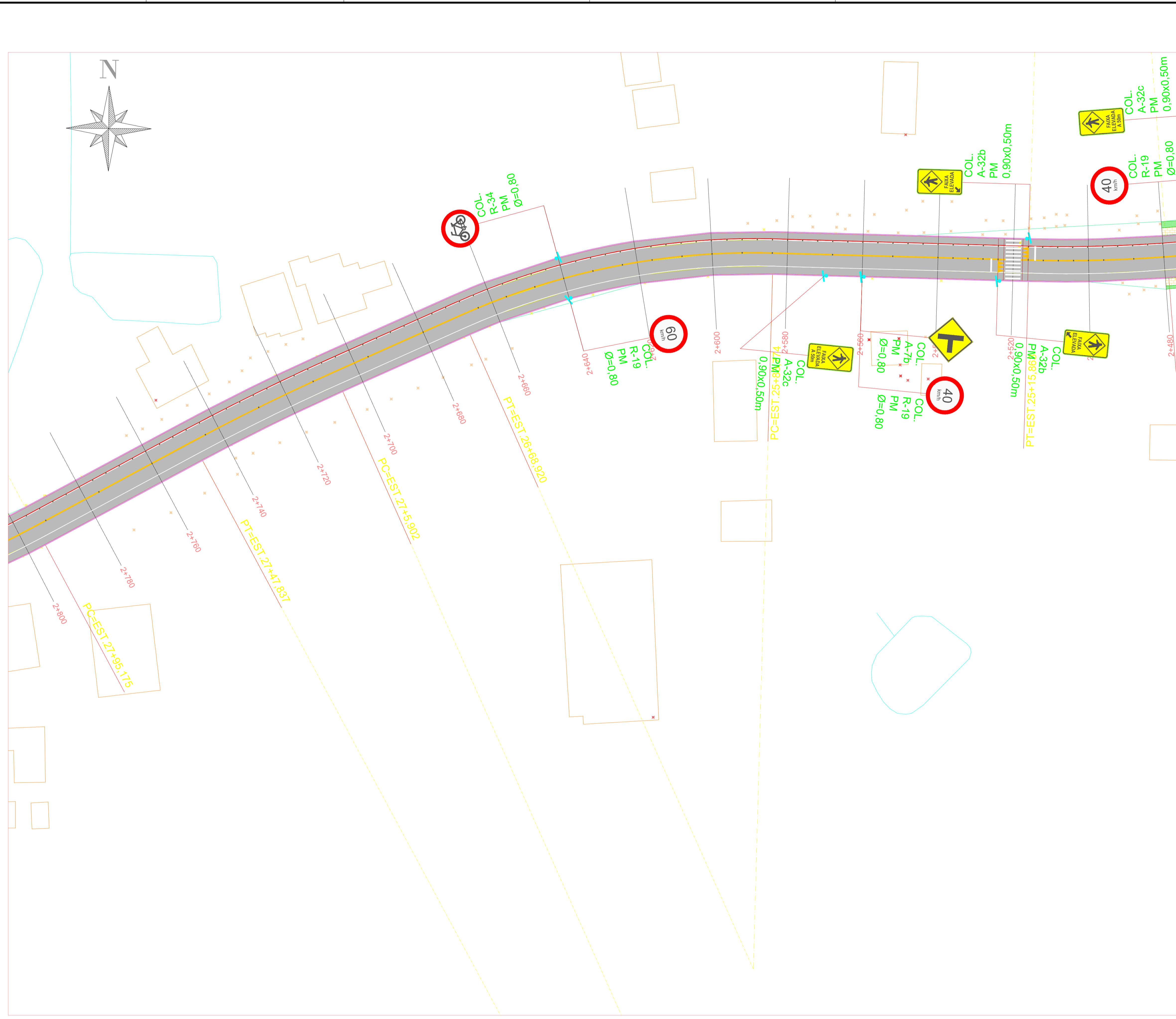
PLANTA BAIXA ESTACA 2+480 A 2+800 ESC: 1/500
