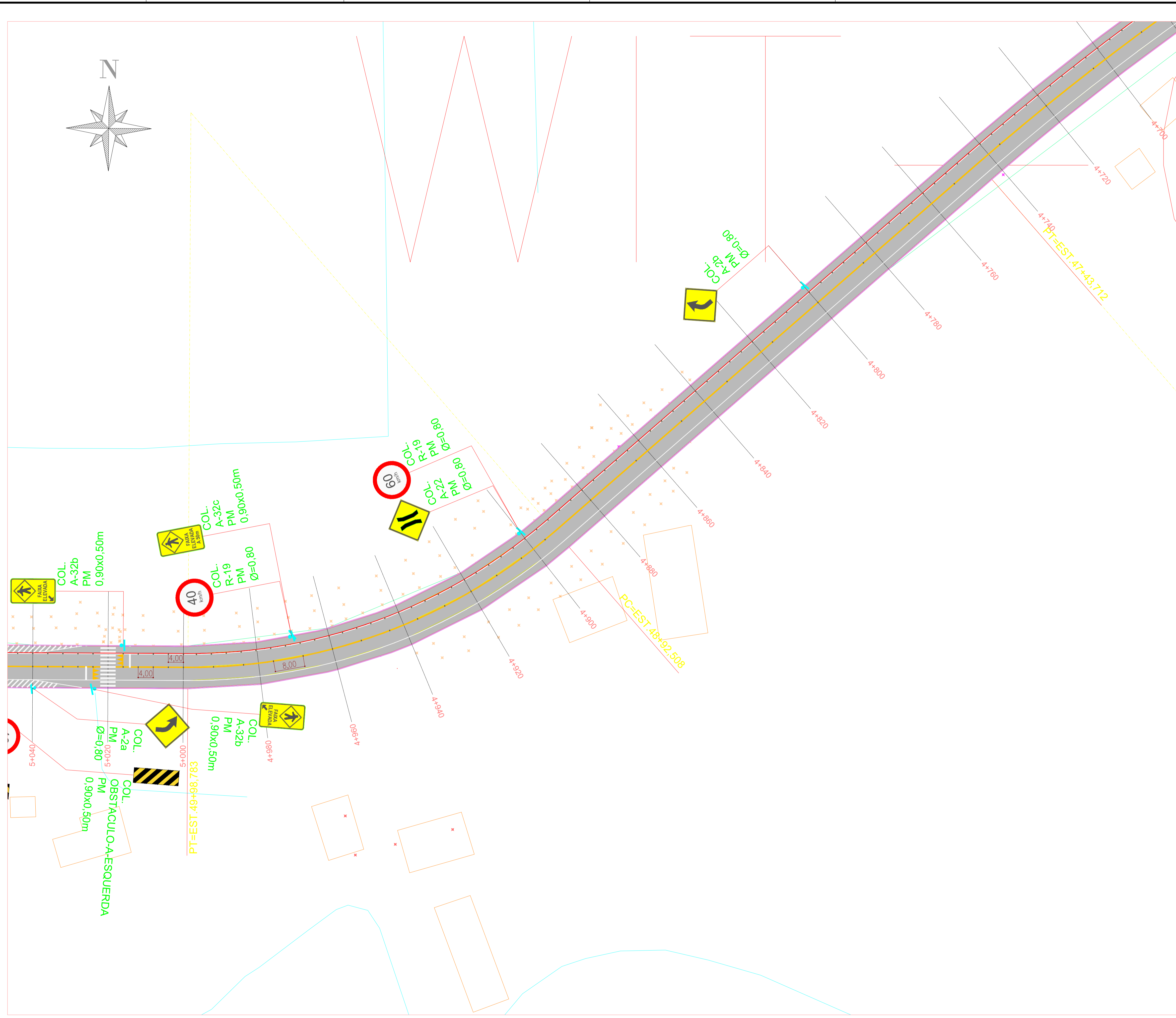
PLANTA BAIXA ESTACA 4+700 A 5+040 ESC: 1/500
