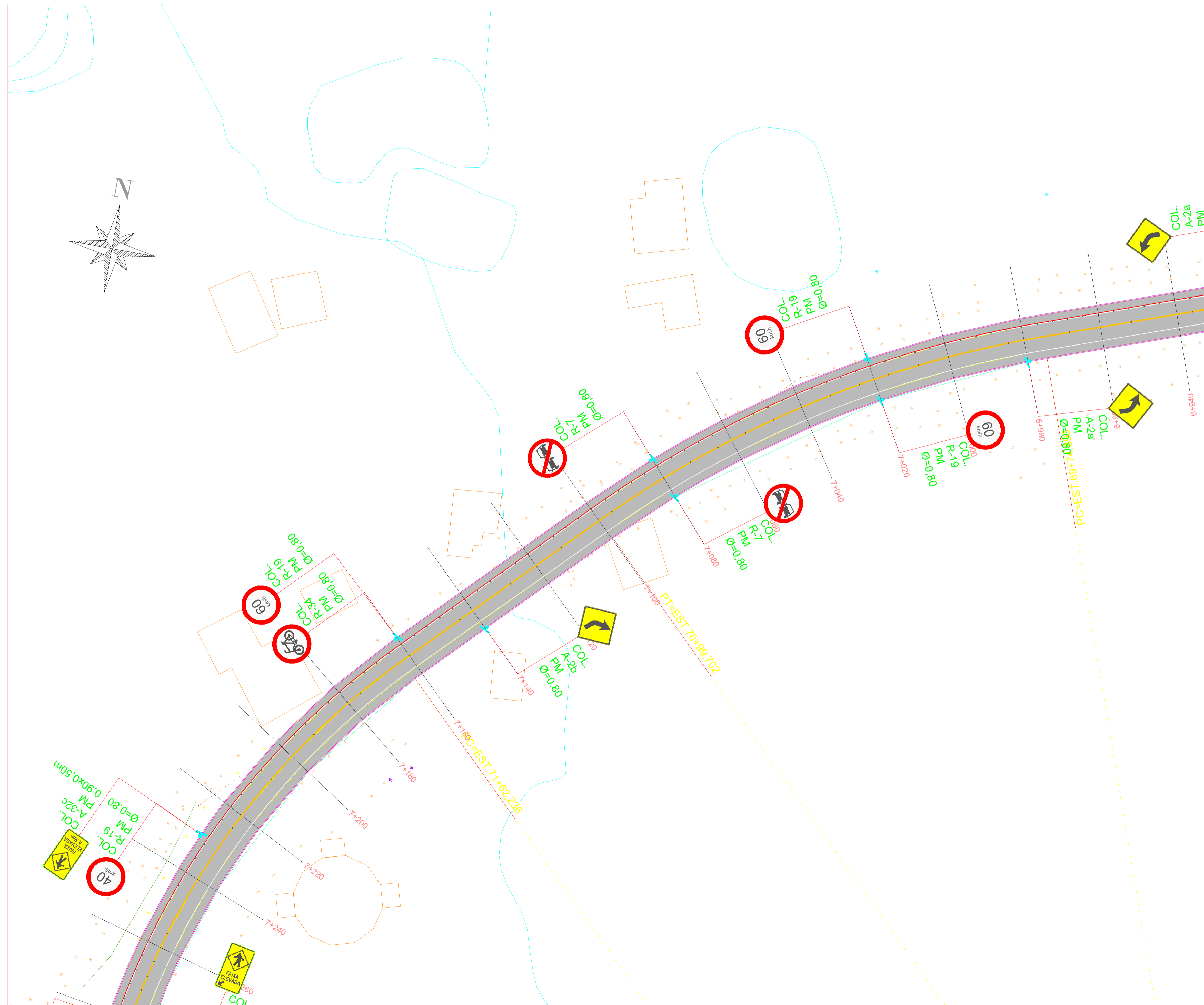
PLANTA BAIXA ESTACA 6+940 A 7+260 ESC: 1/500
