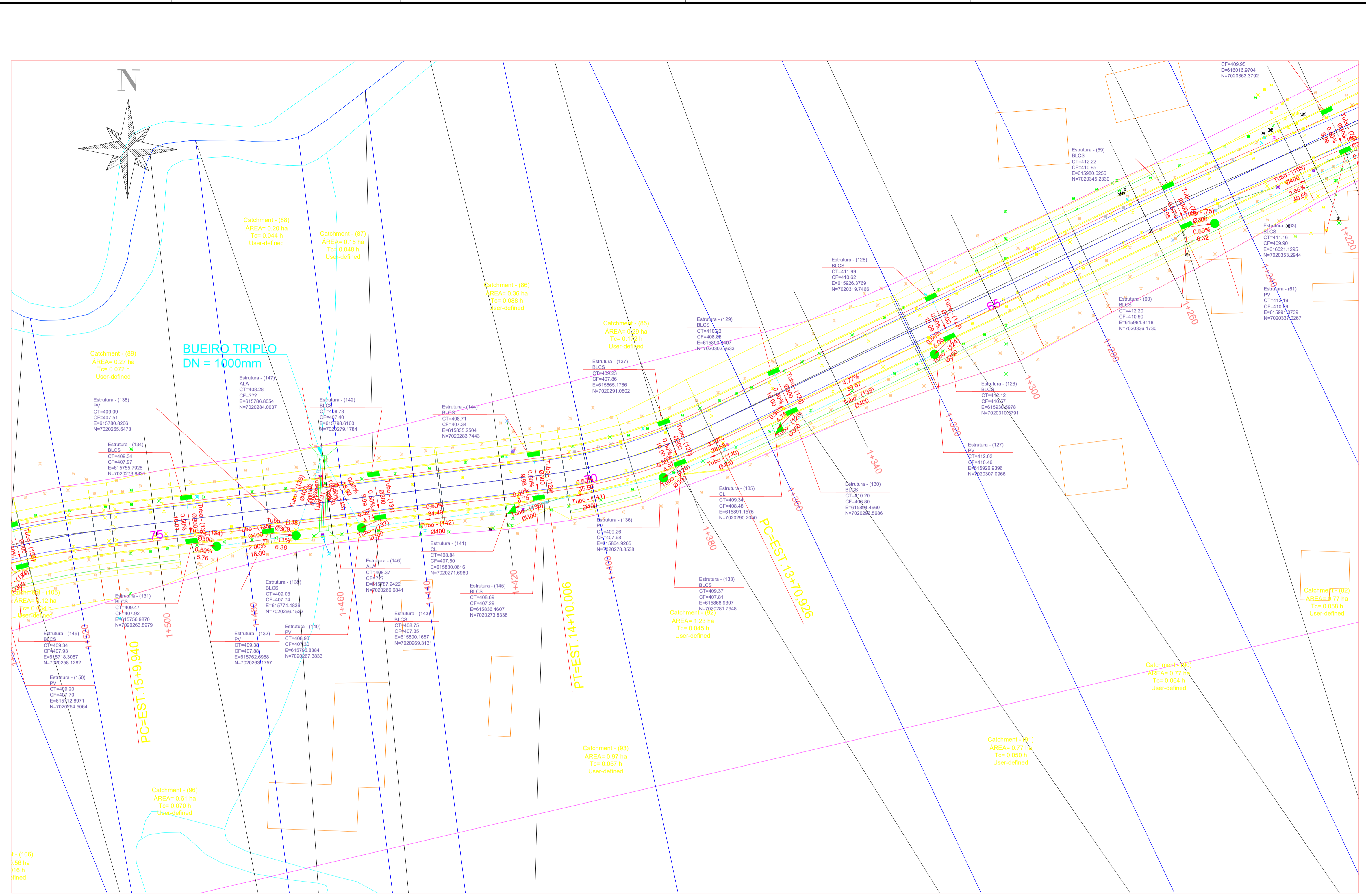
PLANTA BAIXA ESTACA 1+220 A 1+520 ESC: 1/500
