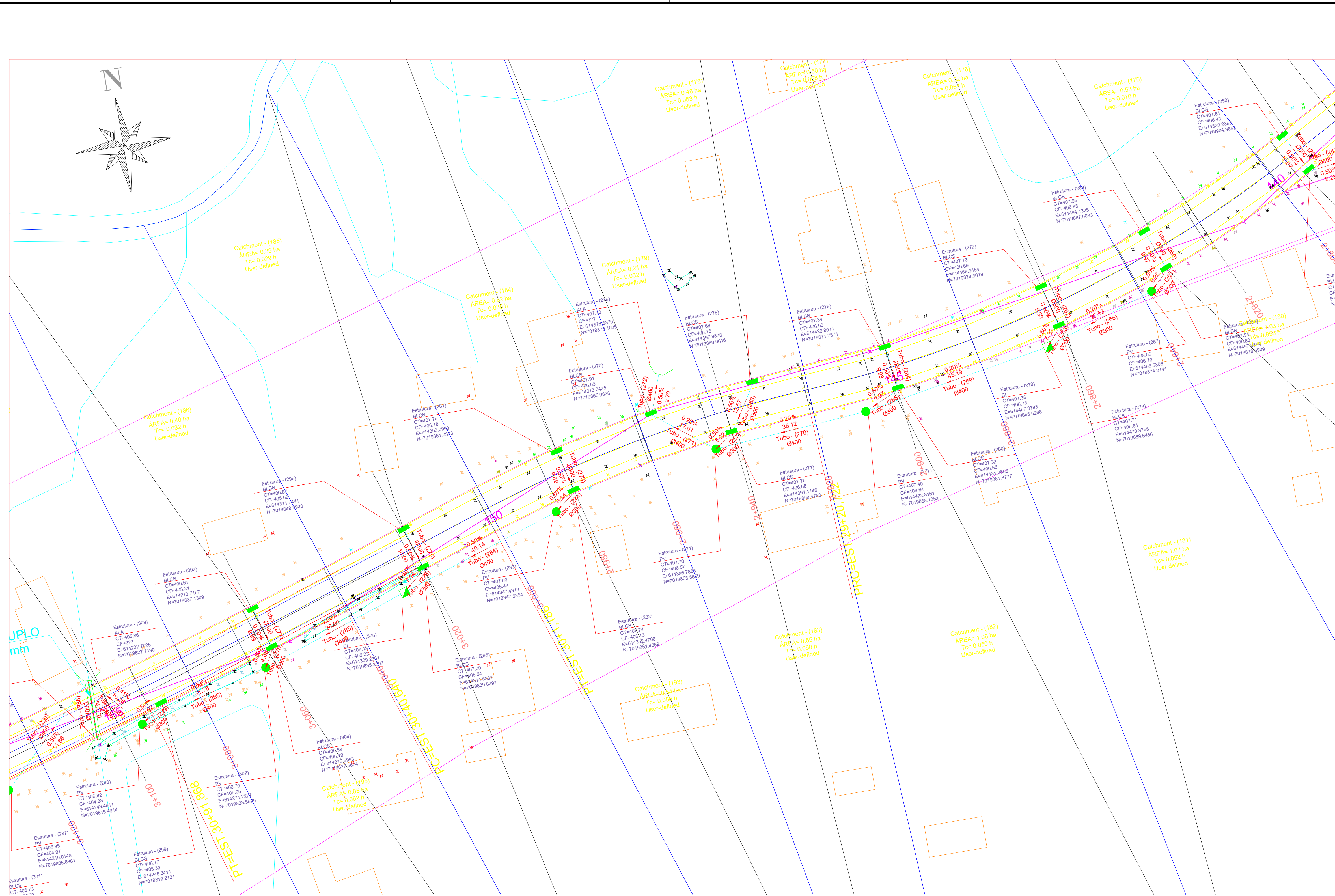
PLANTA BAIXA ESTACA 2+800 A 3+120 ESC: 1/500
