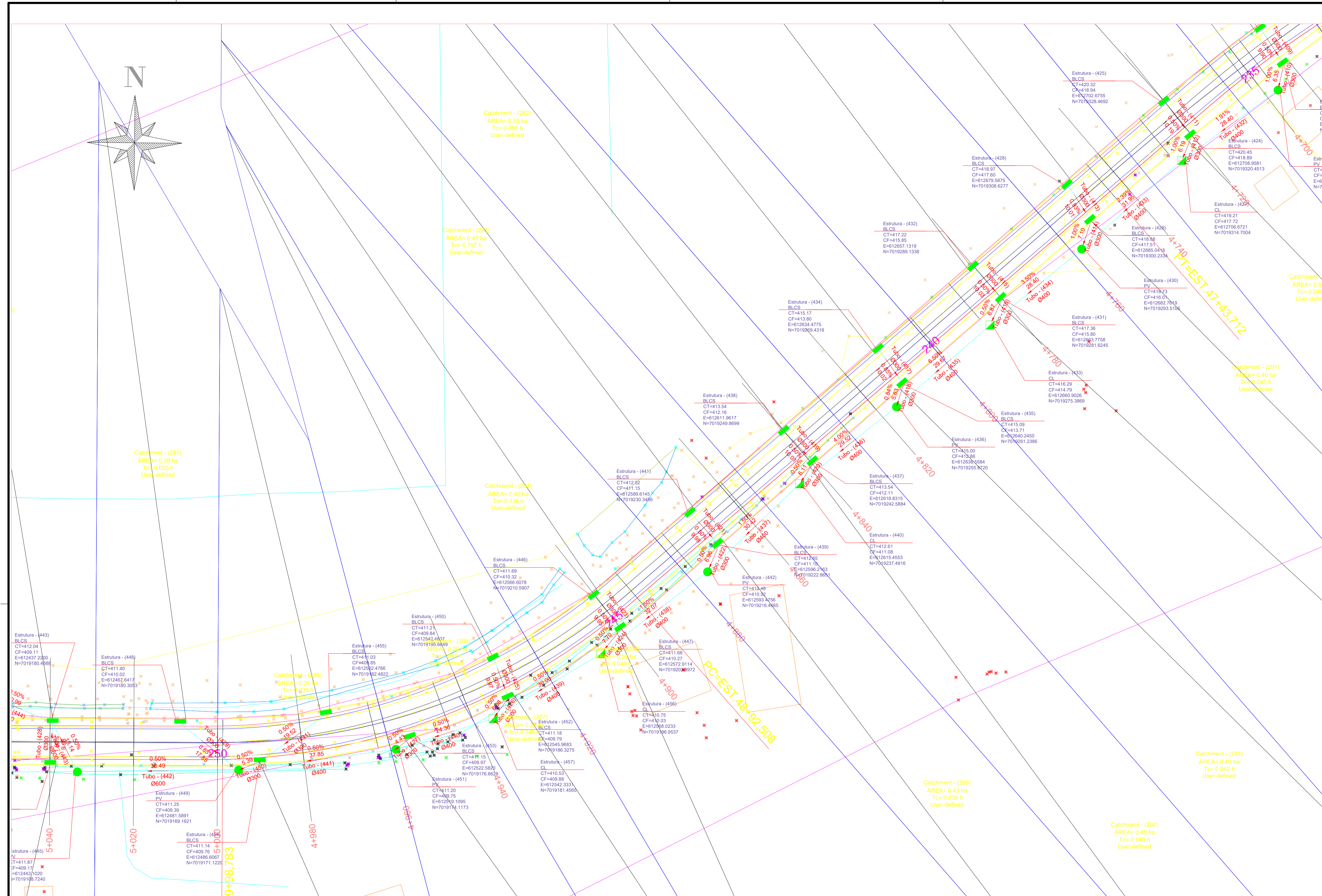
PLANTA BAIXA ESTACA 4+700 A 5+040 ESC: 1/500
