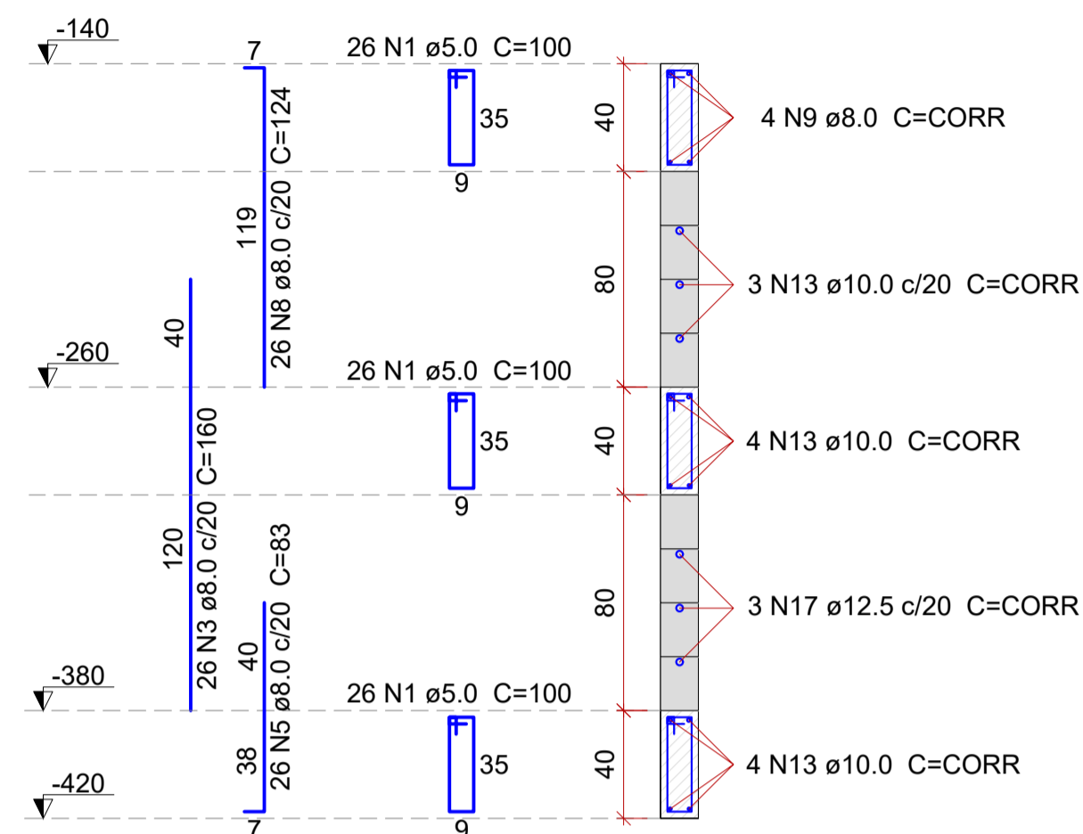
PAR2-PAR5 ESC.: 1:25
