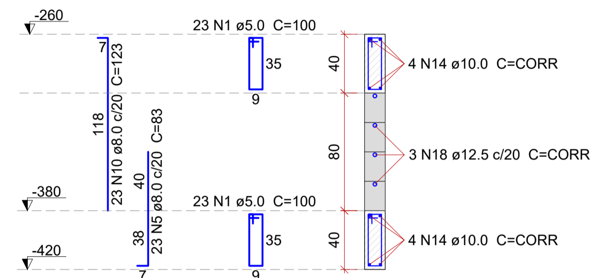
PAR3-PAR6 ESC.: 1:25
