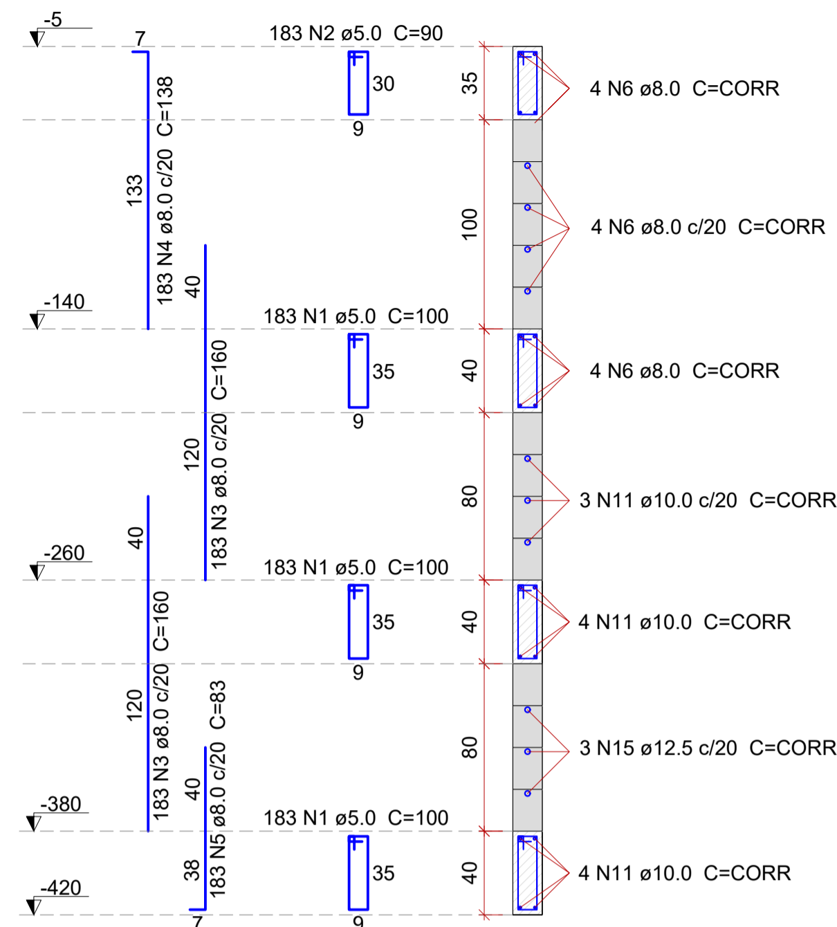
PAR1-PAR4 ESC.: 1:25
