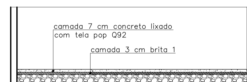
PROJETO PISO CONCRETO
