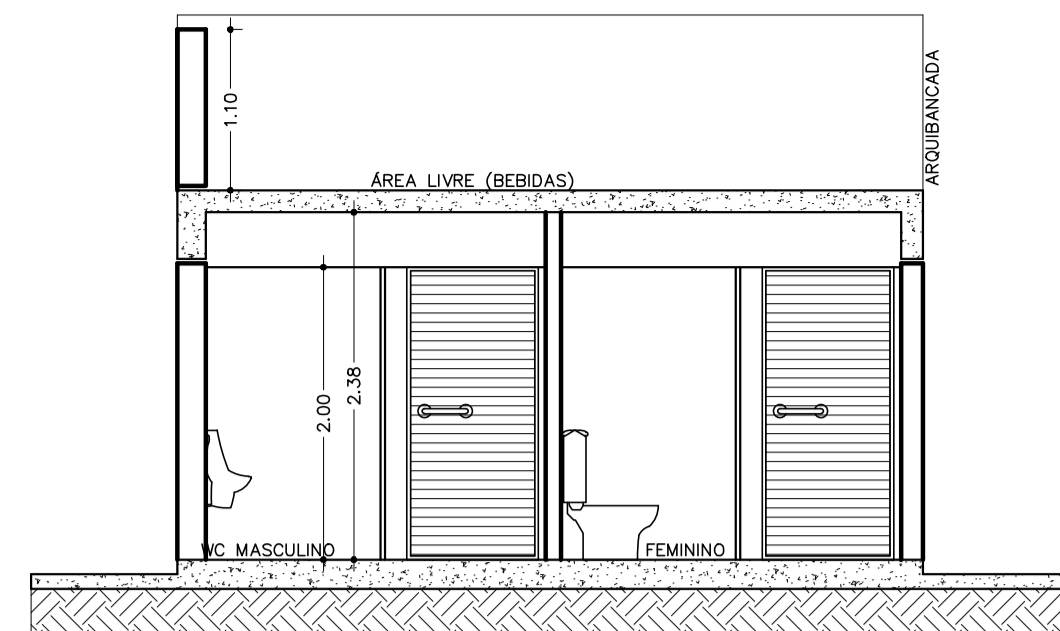
CORTE A-A
