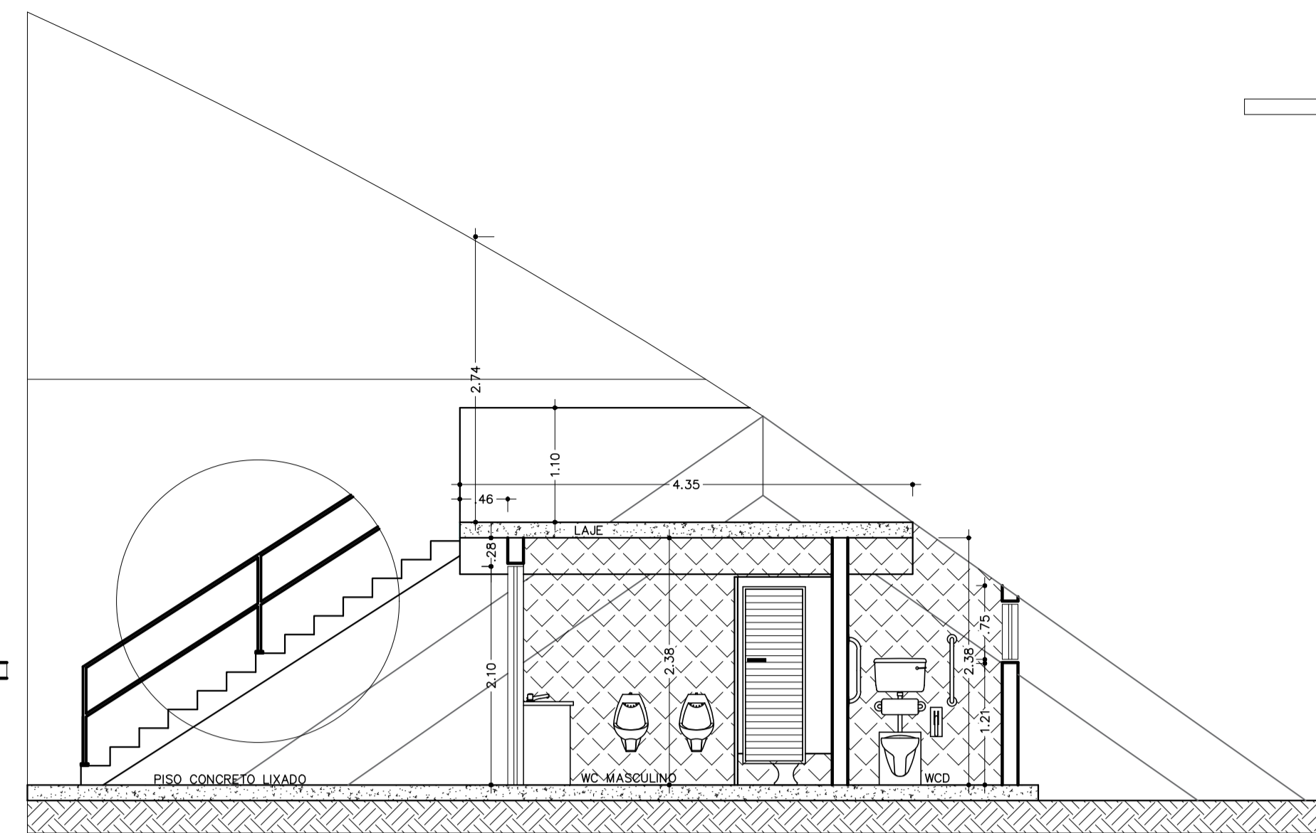
CORTE B-B
