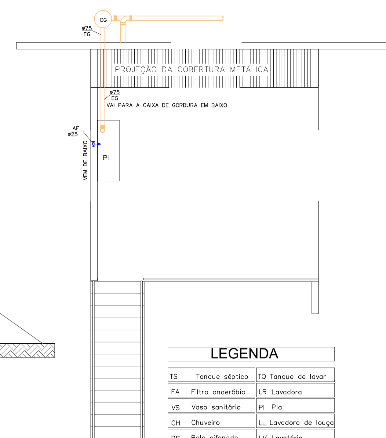
PROJETO ÁGUA TRATADA ESGOTO
