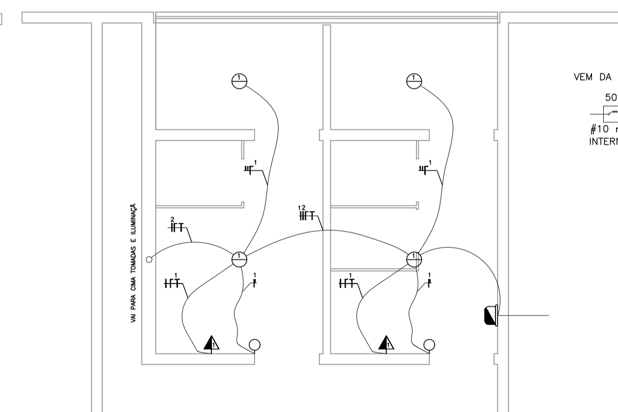
PROJETO ELÉTRICO BANHEIROS
