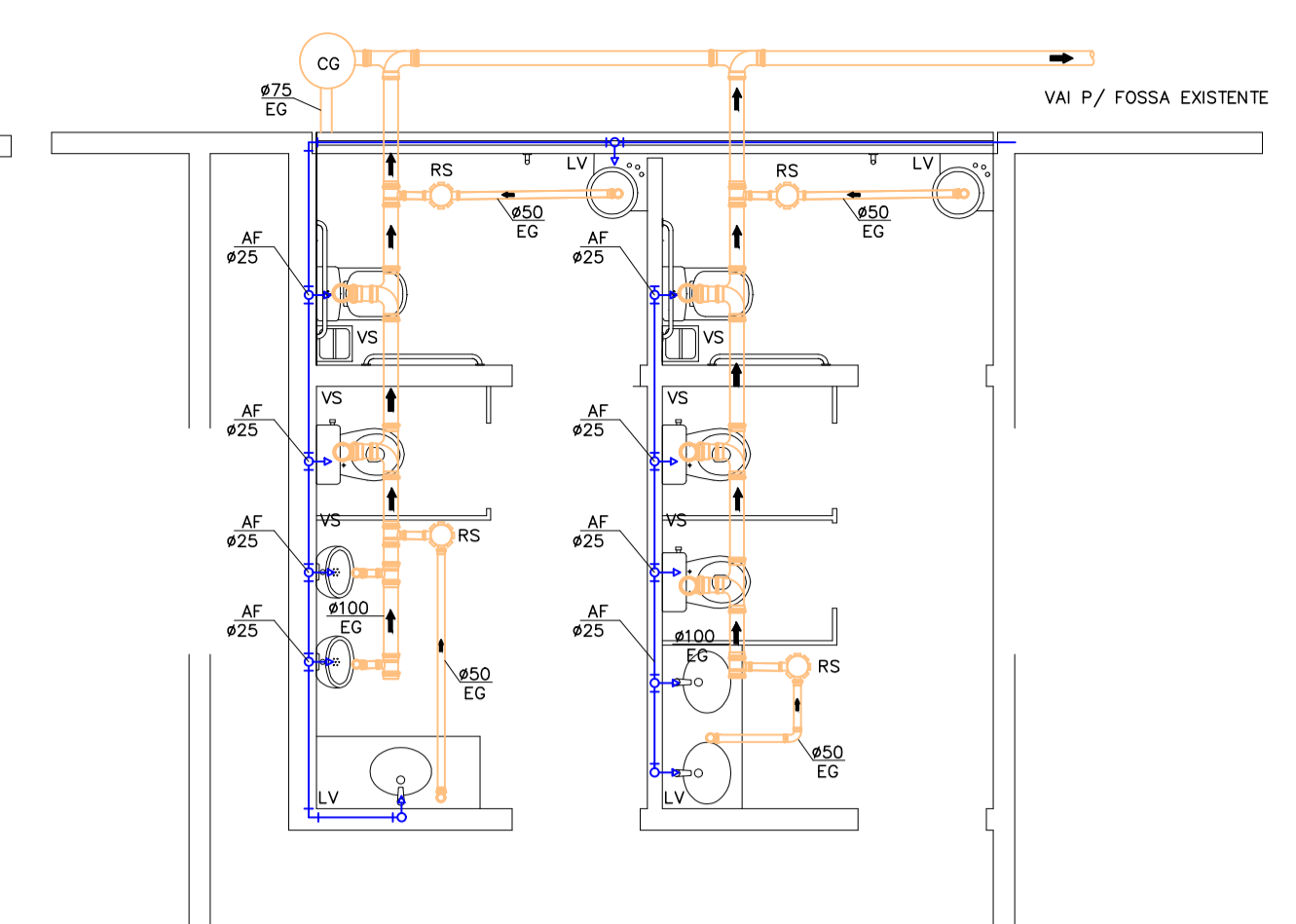
PROJETO ÁGUA TRATADA ESGOTO
