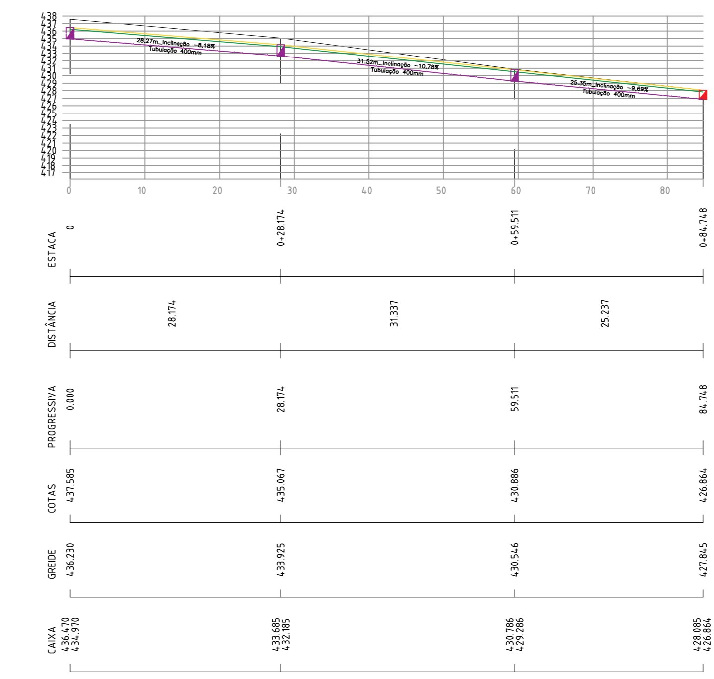
PERFIL DA DRENAGEM Rua Lídia Paduin Escala : 1/500
