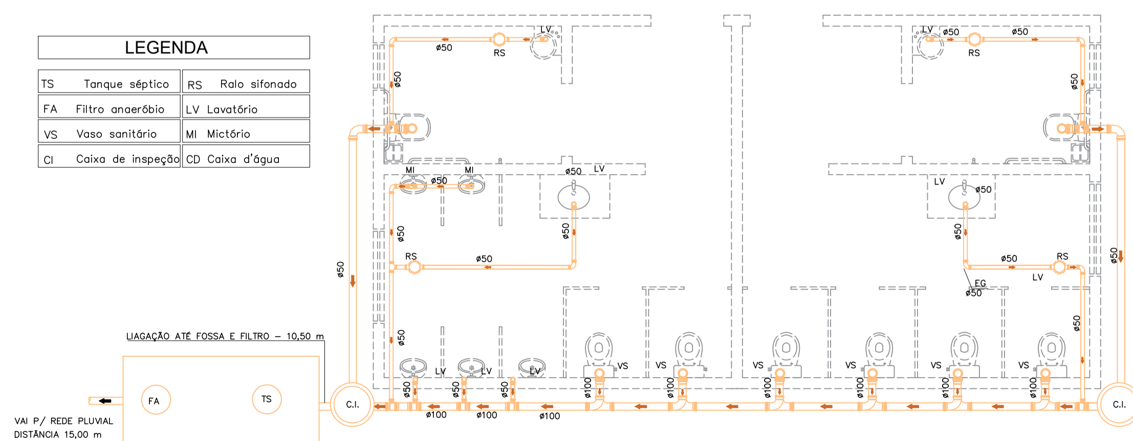
PROJETO ESGOTO Escala : 1/50
