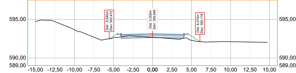
Seção: 09 8+6,30m
