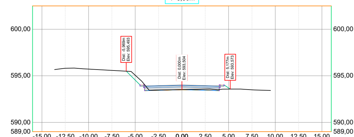
Seção: 04 4+6,30m
