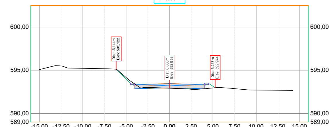
Seção: 07 7+0,00m
