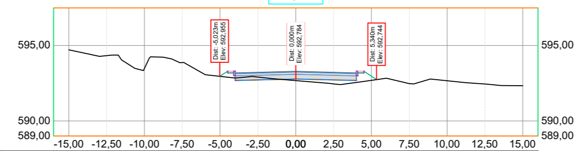
Seção: 08 8+0,00m
