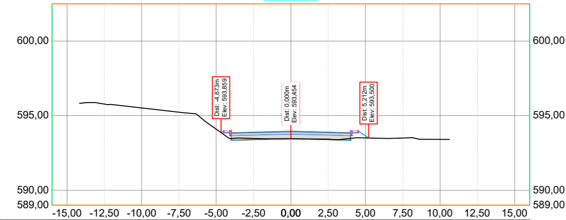
Seção: 05 5+0,00m
