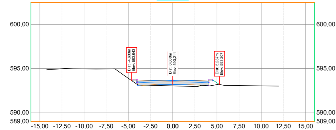
Seção: 06 6+0,00m
