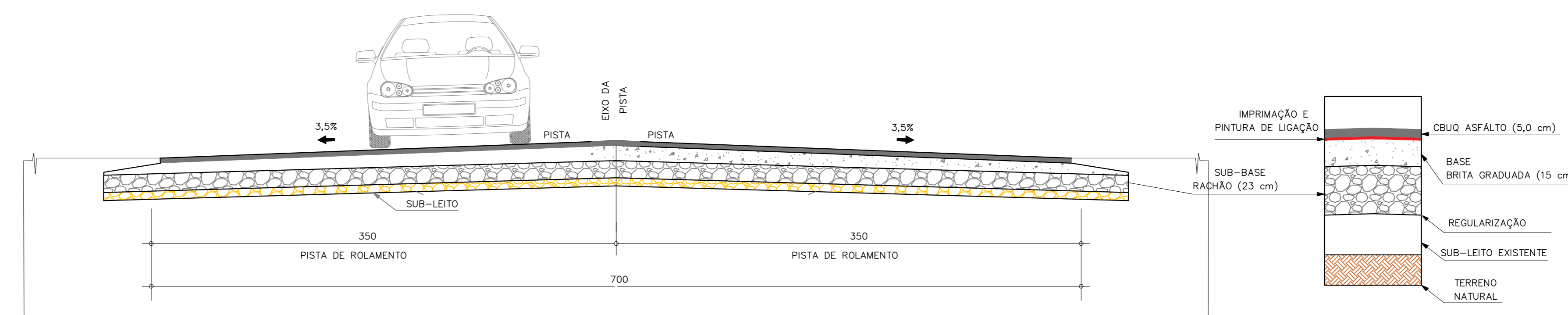
SEÇÃO TIPO - PAVIMENTAÇÃO DA PISTA
